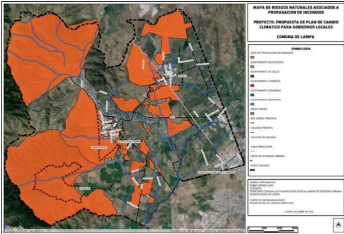
Ilustración 49: Zonas de generación y propagación de incendios según Plan Cambio Climático Lampa 196
